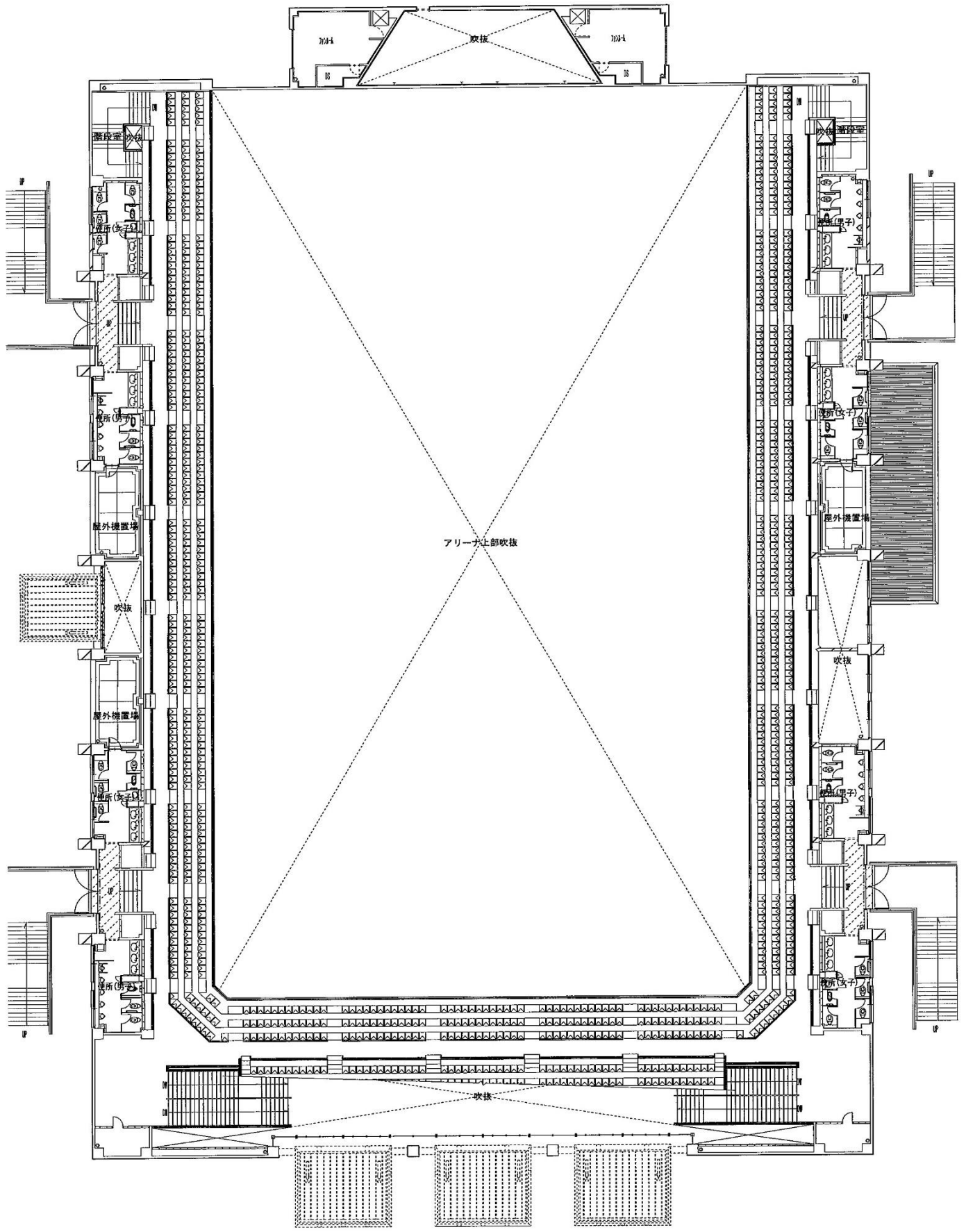
2階平面図
